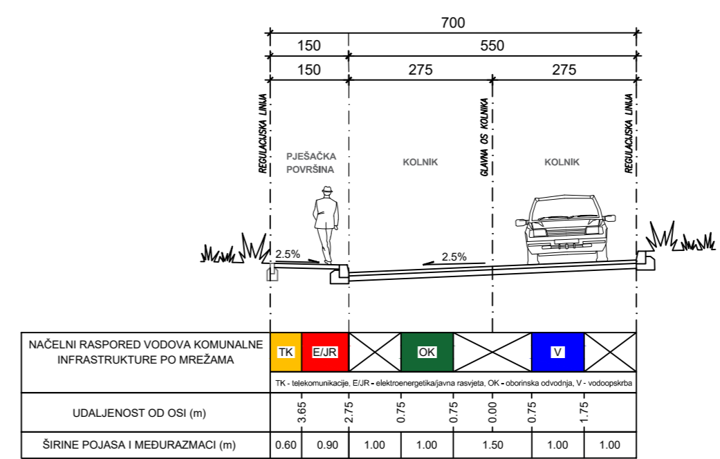
JAVNA PRISTUPNA PROMETNICA (IS4) - PRESJEK - M.J. 1:100
